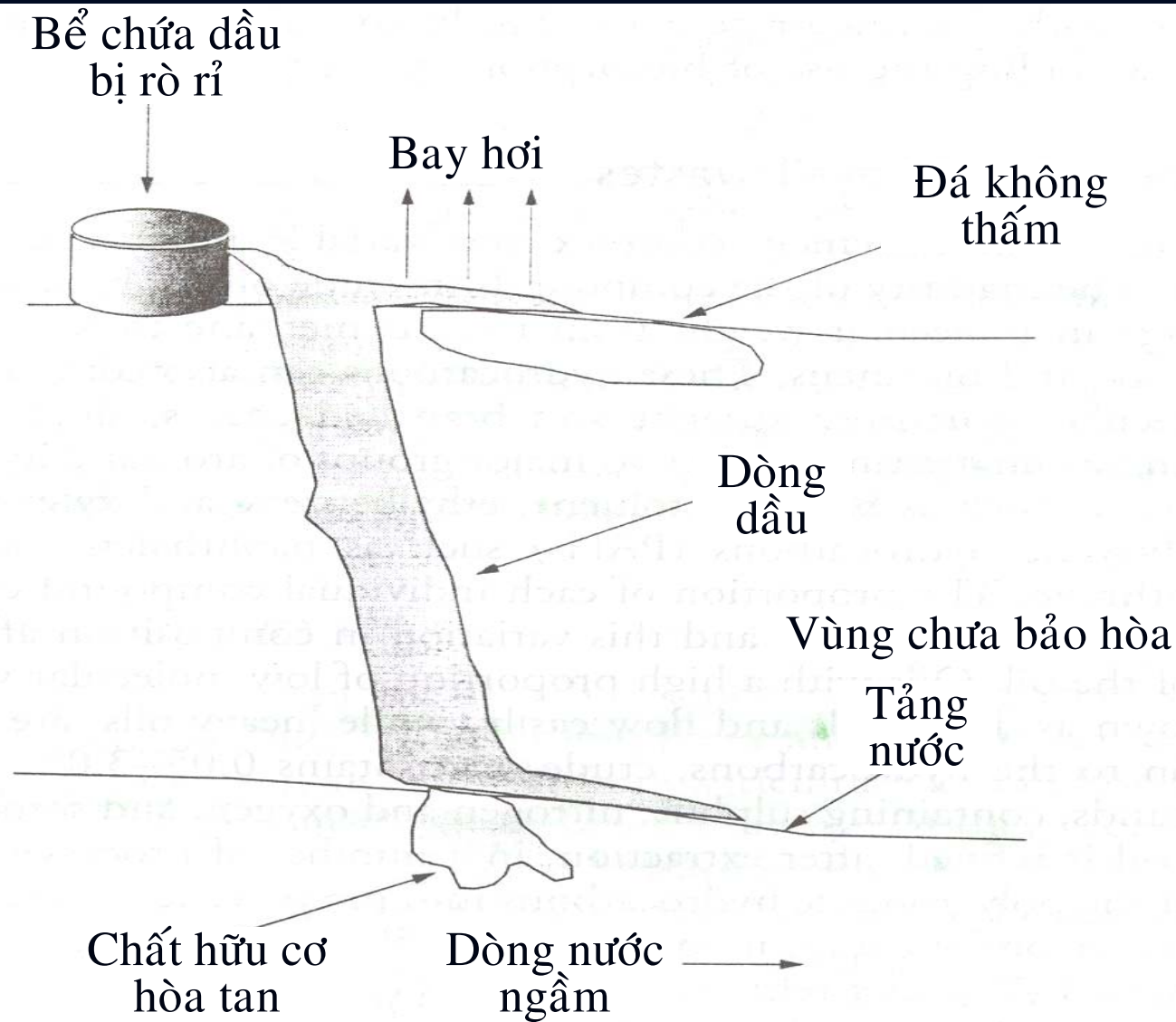
Sự phân bố hydrocarbon trong đất từ sự cố rò rỉ dầu (Bossert và Compeau, 1995)
