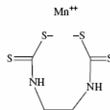
Maneb
